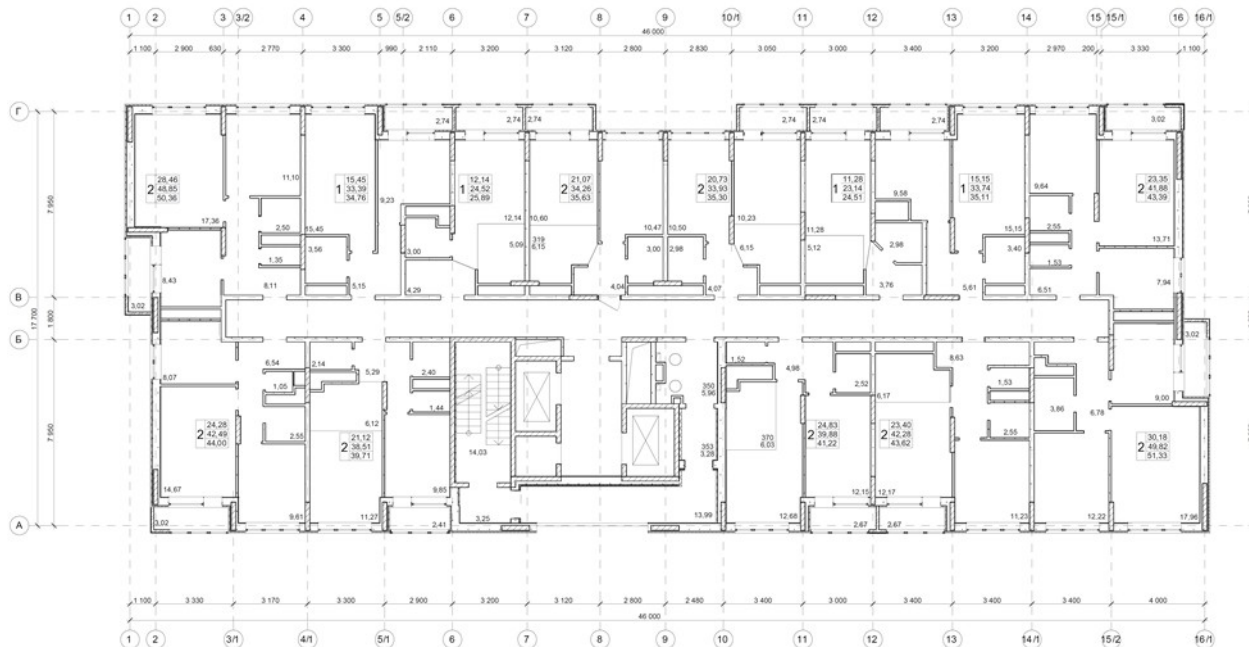
План типового этажа на отм.+6,900...+33,900
